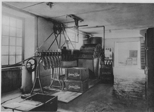
Depot Solothurn, Flaschenabfall-Anlage
